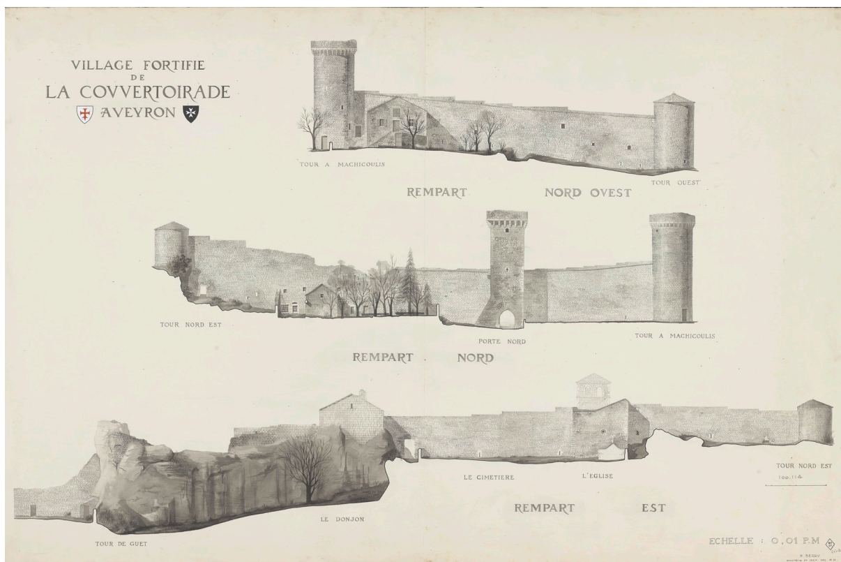
Archive fig. 25 : Élévations des remparts de la Couvertoirade. Dressé par M. Berry, ACMH, 1943. MPP - G/82/12/1004 - 76030.
