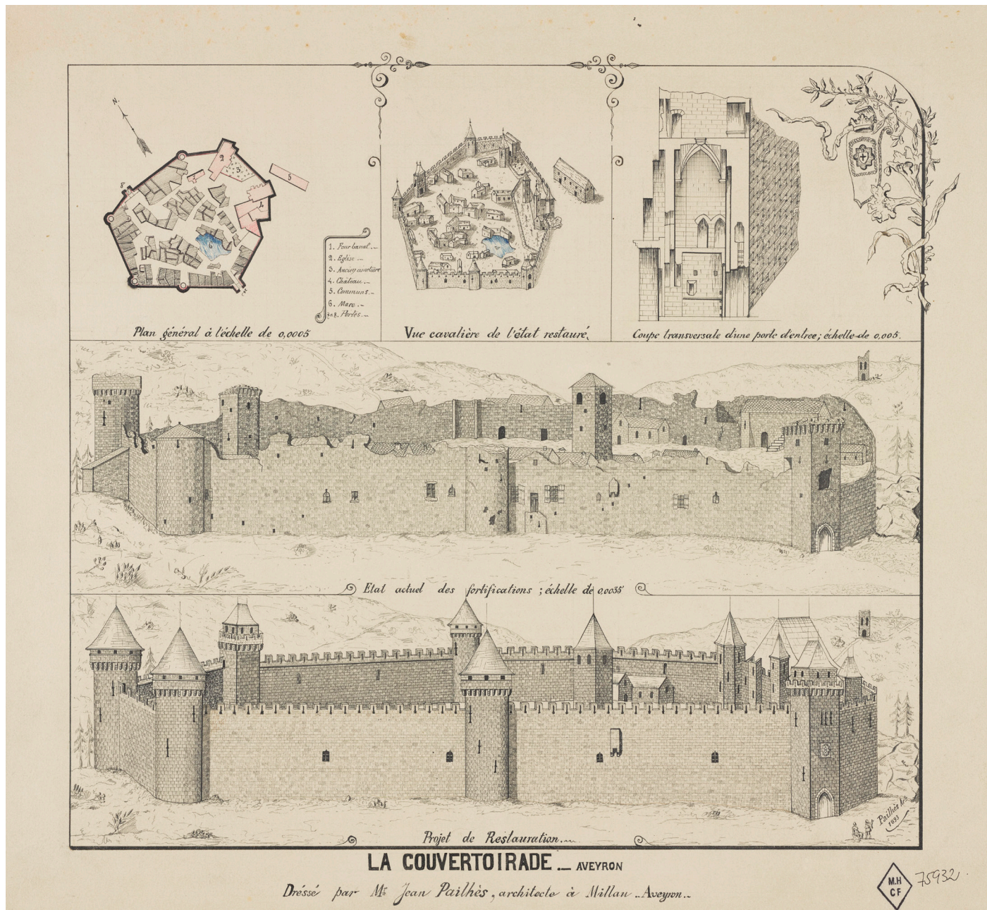
Archive fig. 1 : Plan, axonométrie et élévations de la Couvertoirade représentant un état actuel et un projet de restauration. Dressé par Jean Pailhès, architecte à Millau, 1893. MPP - côte G/82/12/1004 - 75932.
