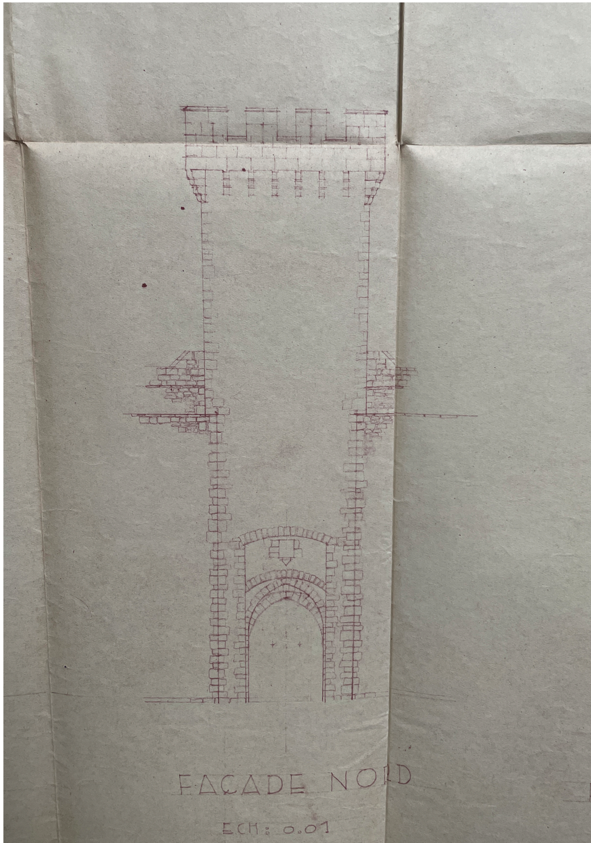
Archive fig. 20 : Extrait de la planche graphique du projet de reconstruction de la tour Sud. Vue de l'élévation Nord. Dressé par M. Berry, ACMH, 1941. MPP - côte E/81/12/7-46.
