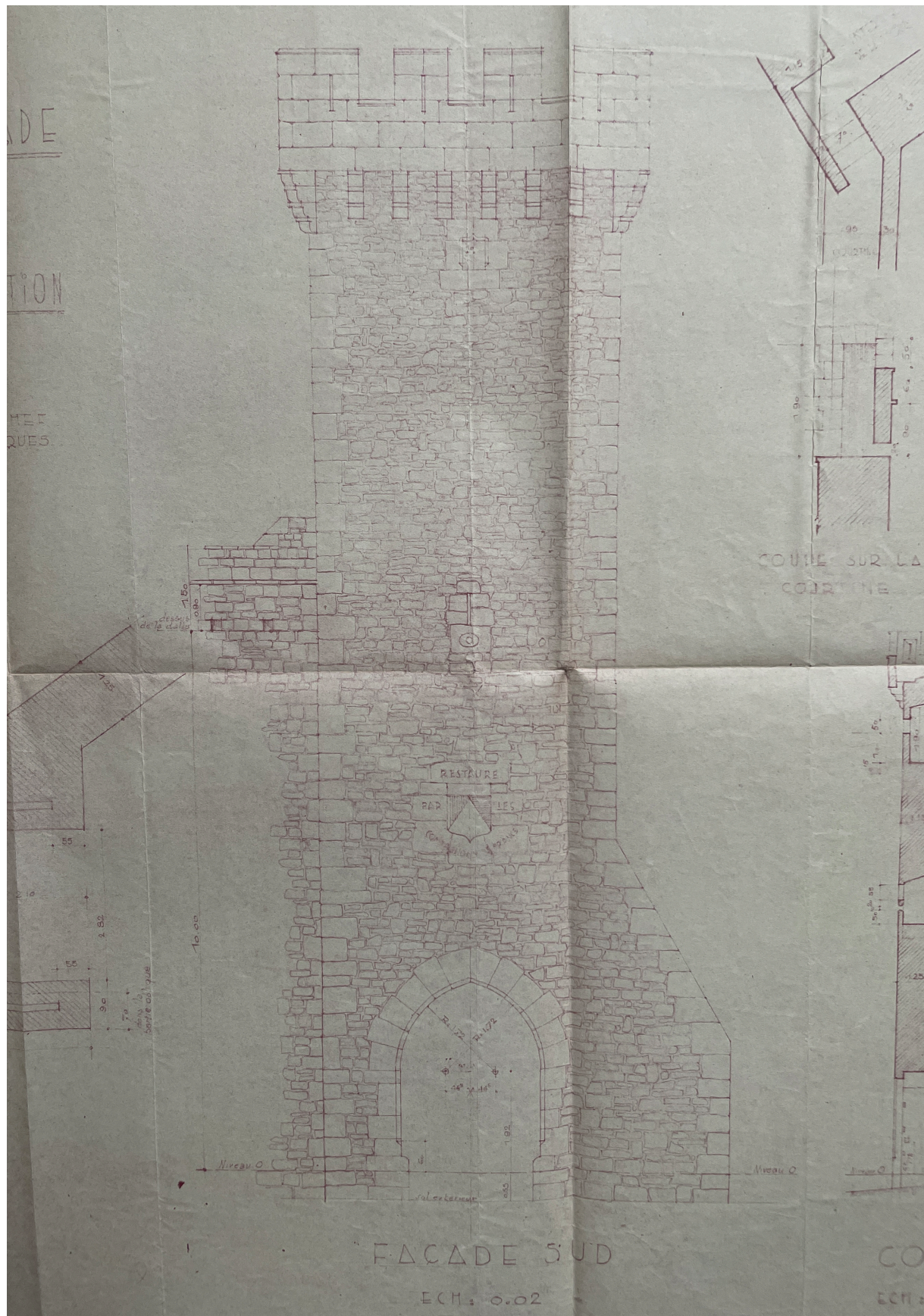
Archive fig. 19 : Extrait de la planche graphique du projet de reconstruction de la tour Sud. Vue de l'élévation Sud. Dressé par M. Berry, ACMH, 1941. MPP - côte E/81/12/7-46.
