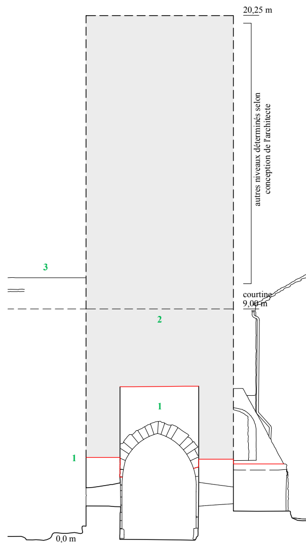
COUPE
