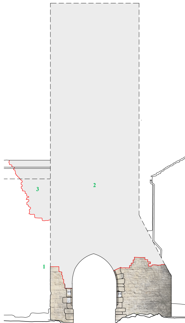
ELEVATION SUD
