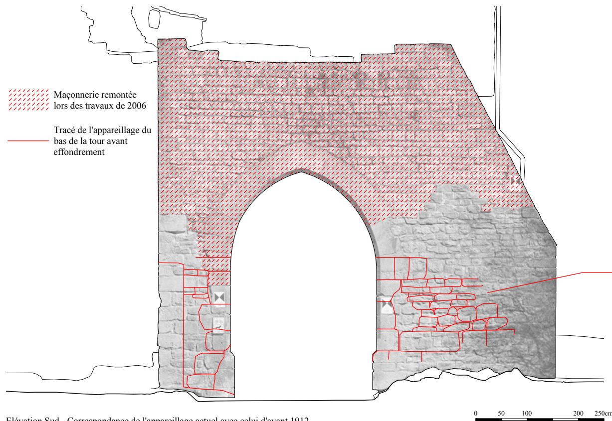
Elévation Sud - Correspondance de l'appareillage actuel avec celui d'avant 1912.
