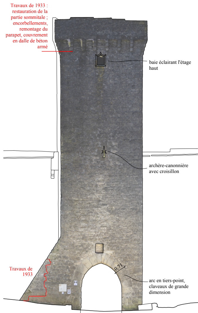
ELEVATION NORD
