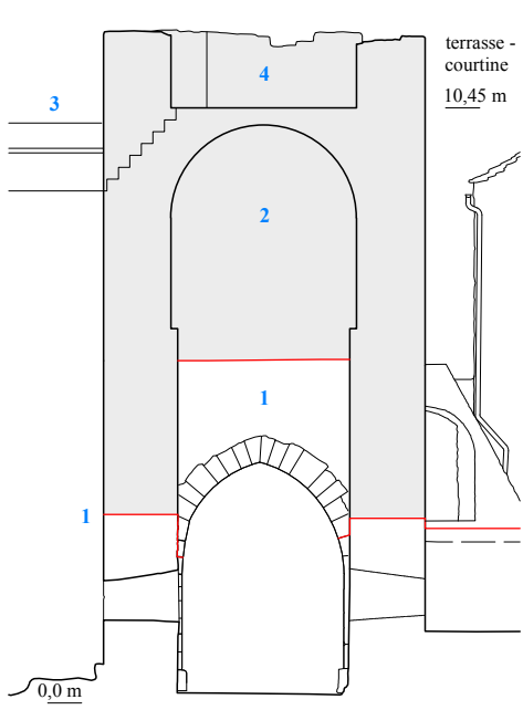
COUPE
