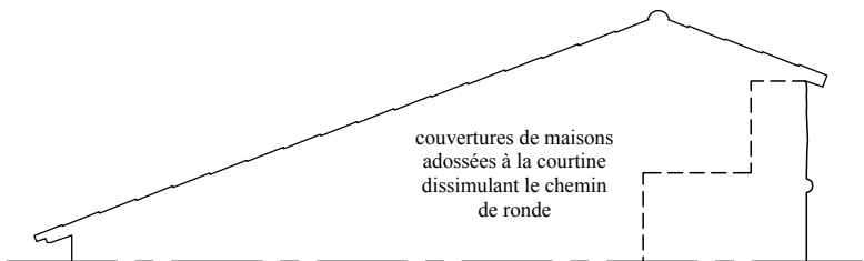
COUPE
