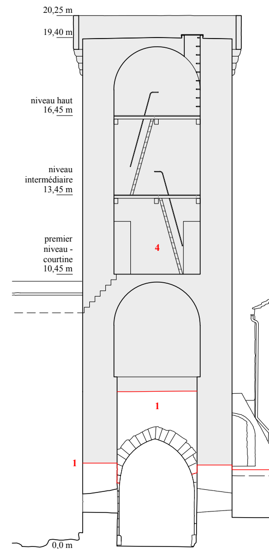
COUPE EST-OUEST
