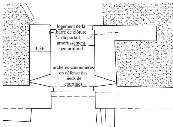
PLAN DU REZ-DE-CHAUSSEE
