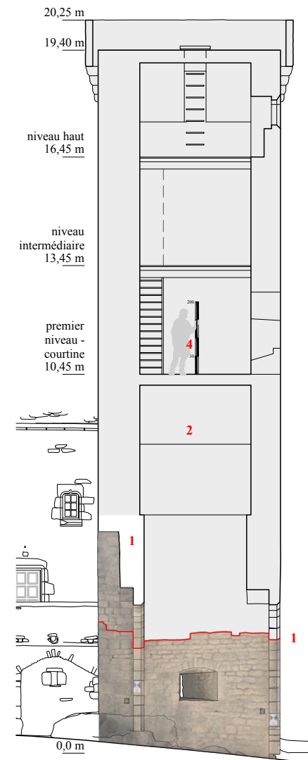
COUPE NORD-SUD
